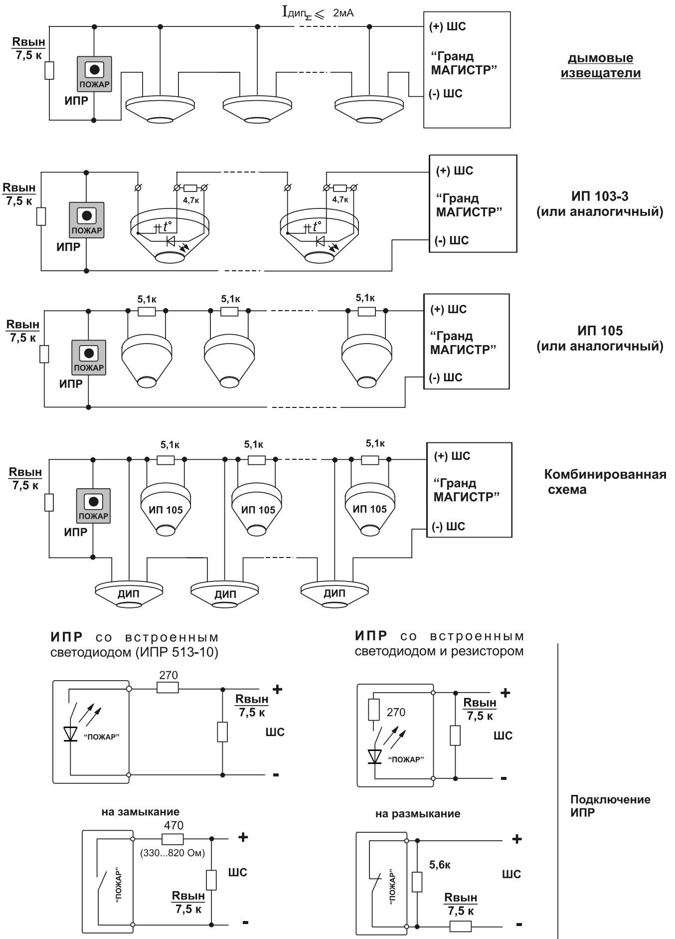
Рис. 7. Организация однопорогового шлейфа пожарной сигнализации
