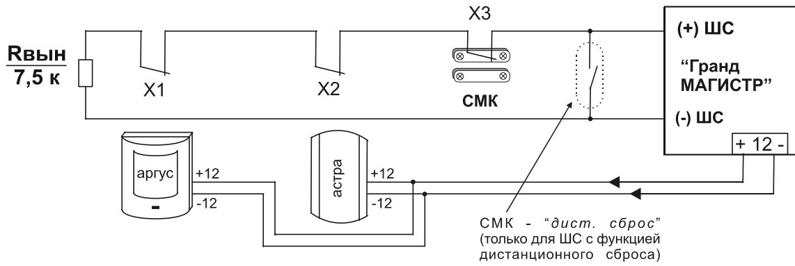
Рис. 8. Схема подключения ШС с охранными извещателями
